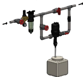
Instalación bypass
