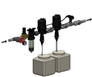
Installation avec double injection à distance
