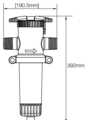
Dimensiones filtros 1.5"
